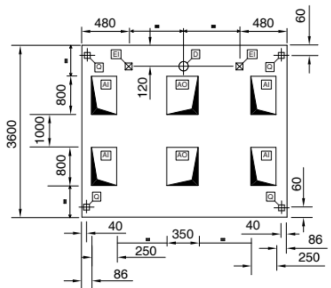
Top
