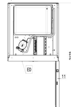
Top
