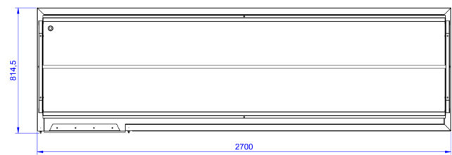
Top
