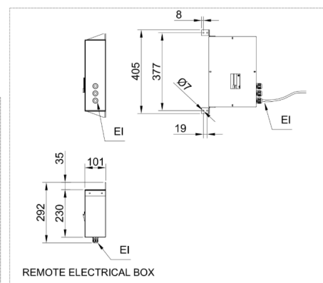
CONTROLLER - 1PC
